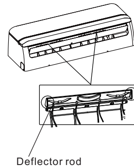
Fig. 11 — Deflector Rod
