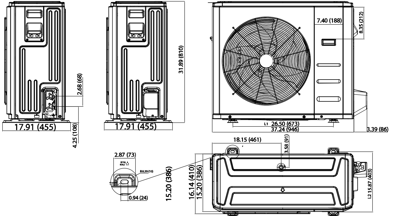
Fig. 1 – Size 36K
