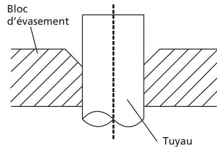
Fig. 14 – Bloc d'évasement
