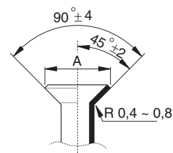
Fig. 15 – Forme évasée
