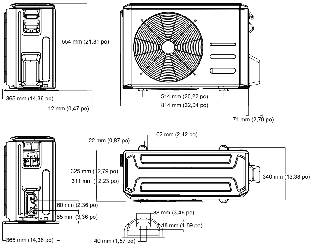
Fig. 4 – Capacités 9K à 12K
