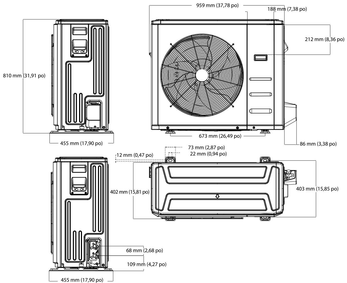
Fig. 6 – Capacités 24K, 30K et 36K
