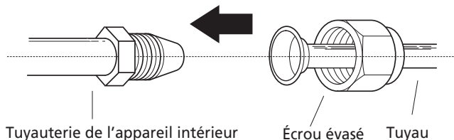
Fig. 16 – Placez le centre des tubes vis à vis.
